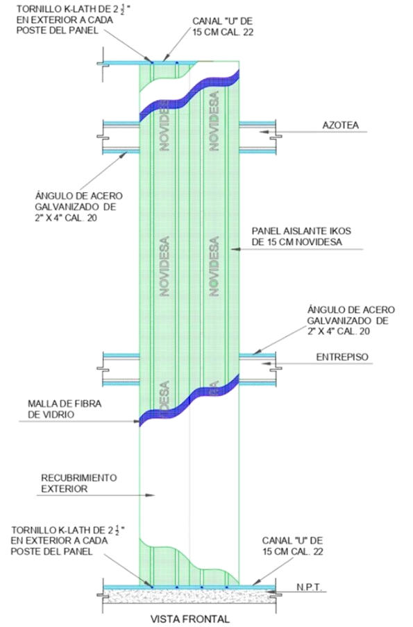
DETALLE DE MURO IKOS CORTINA
