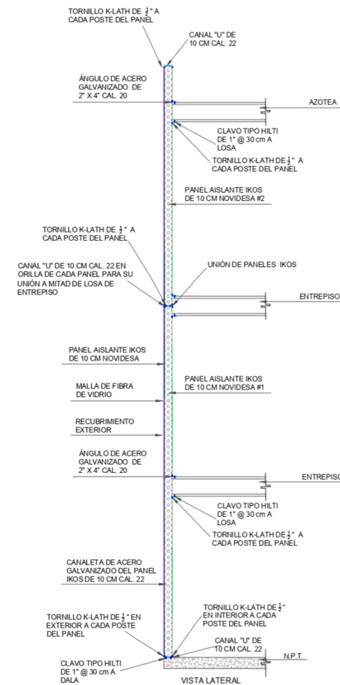
DETALLE DE MURO IKOS CORTINA
