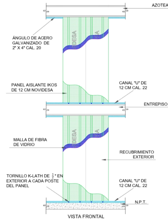
DETALLE DE MURO IKOS TAPÓN
