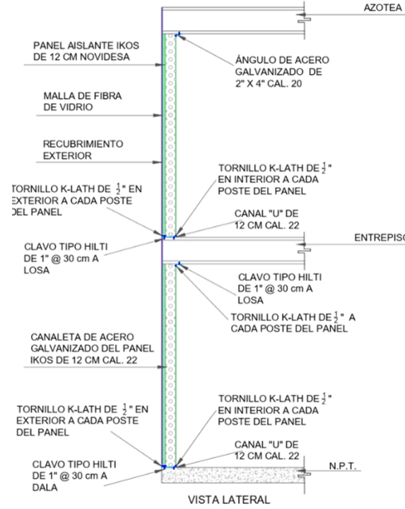
DETALLE DE MURO IKOS TAPÓN
