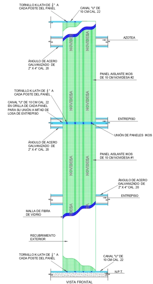
DETALLE DE MURO IKOS CORTINA
