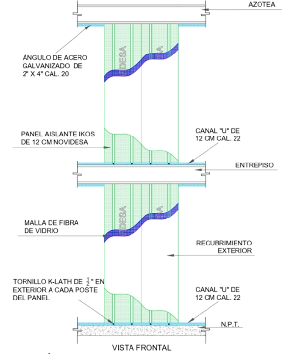
DETALLE DE MURO IKOS TAPÓN
