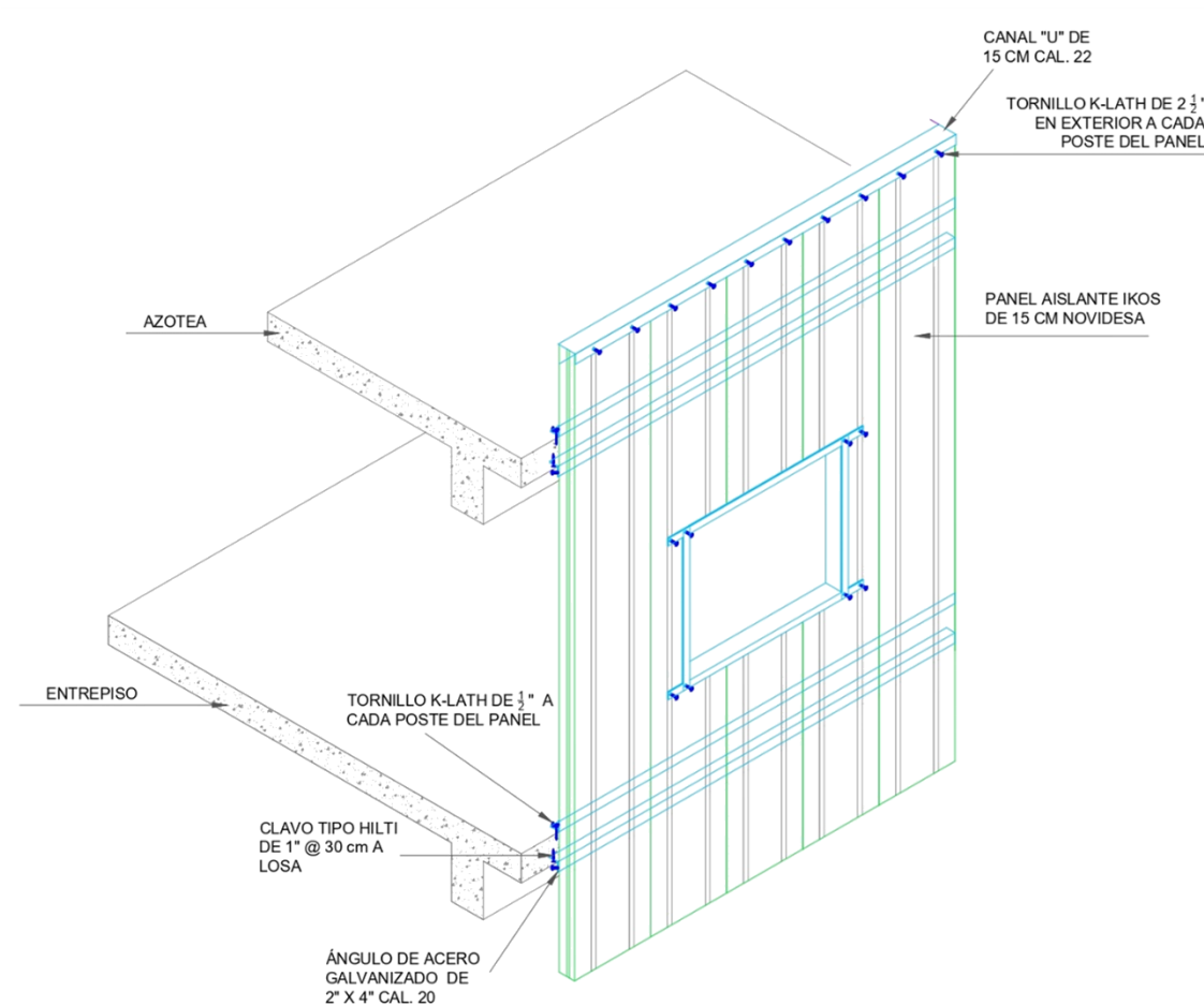
DETALLE IKOS MURO CORTINA
