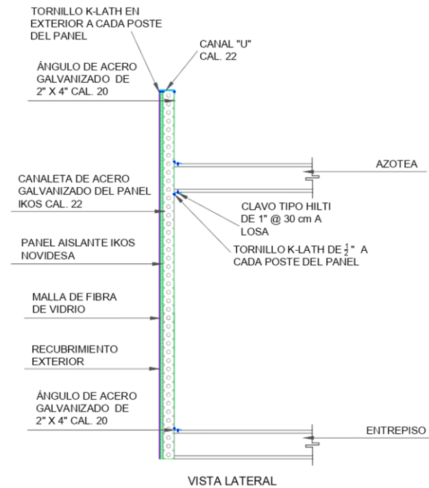
DETALLE DE MURO IKOS CORTINA
