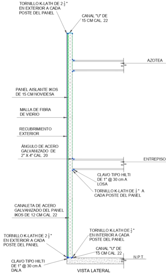
DETALLE DE MURO IKOS CORTINA
