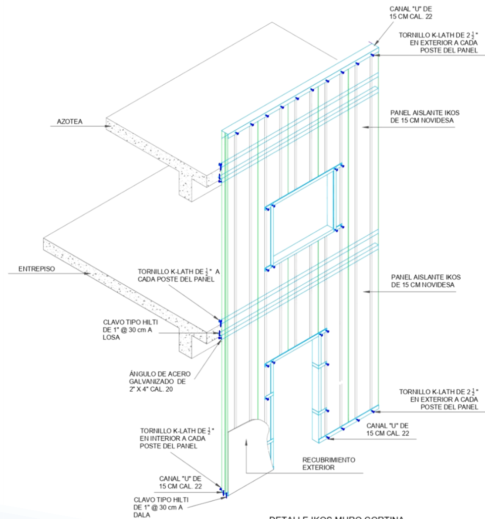
DETALLE IKOS MURO CORTINA
