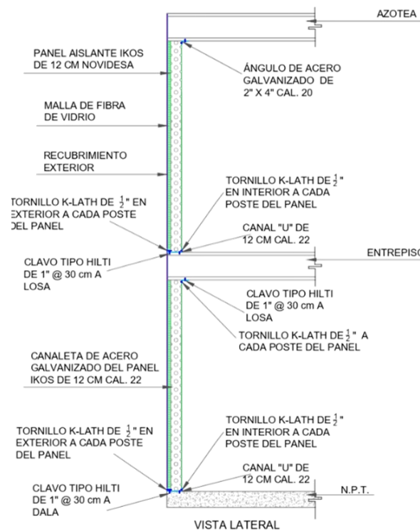
DETALLE DE MURO IKOS TAPÓN
