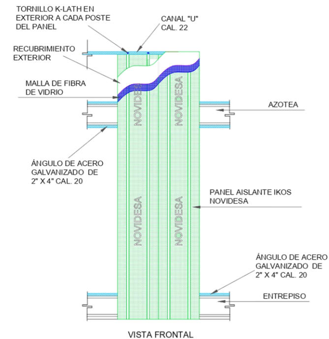
DETALLE DE MURO IKOS CORTINA
