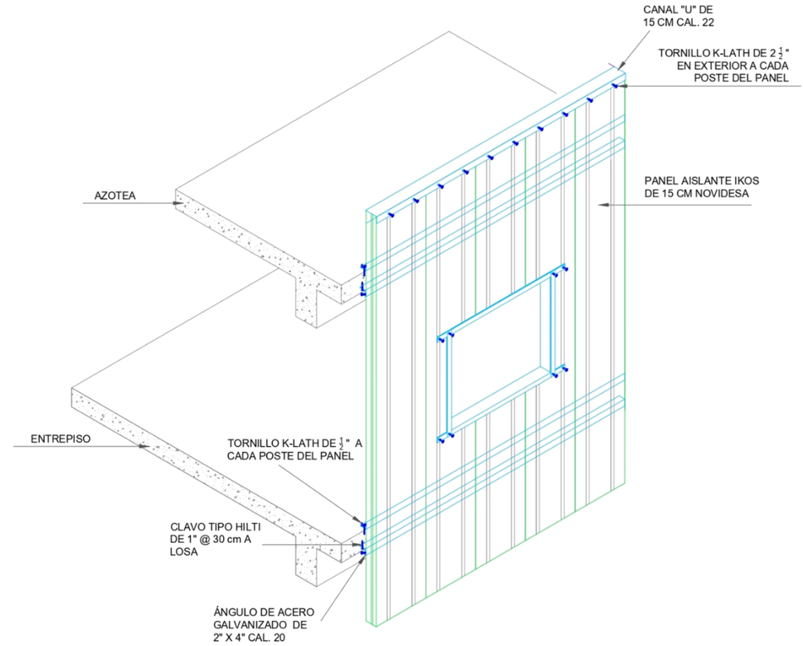
DETALLE IKOS MURO CORTINA
