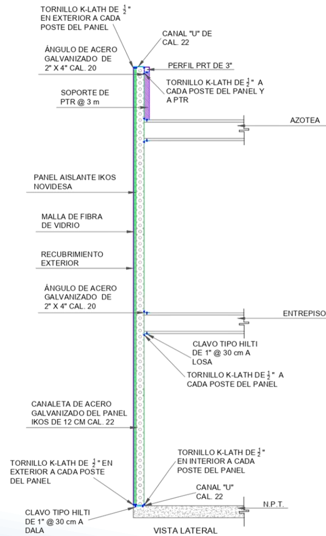
DETALLE DE MURO IKOS CORTINA
