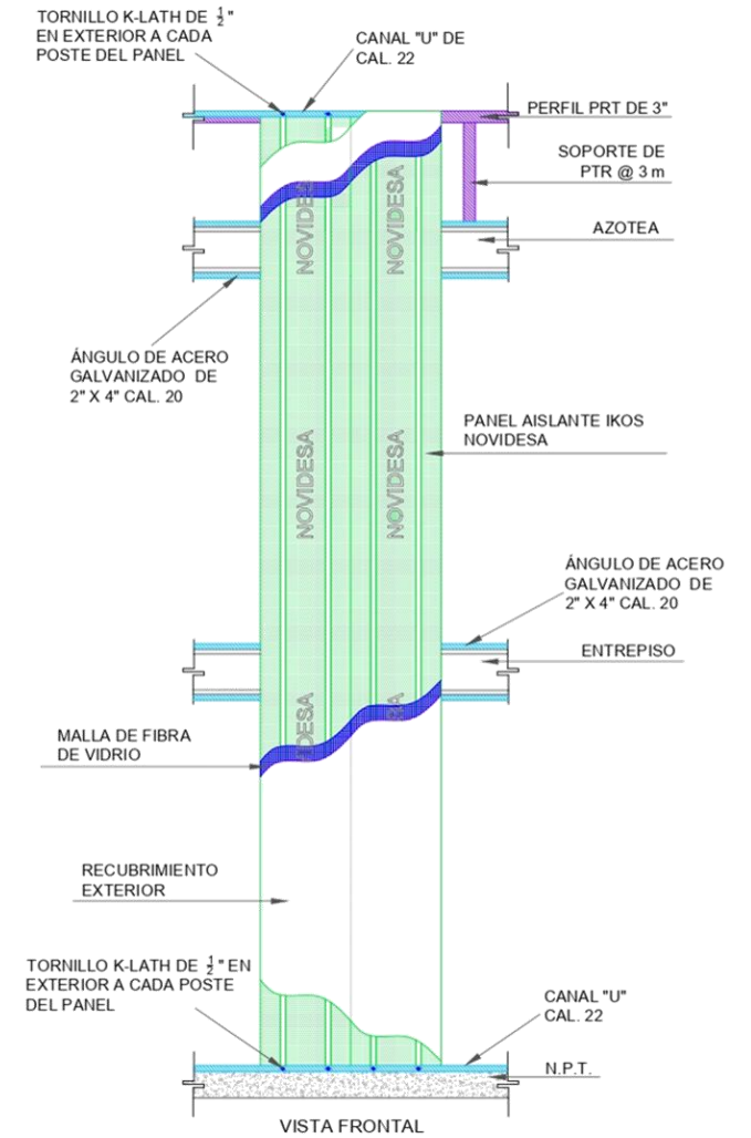
DETALLE DE MURO IKOS CORTINA
